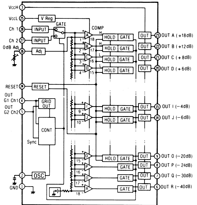
IC501: AN6870N
